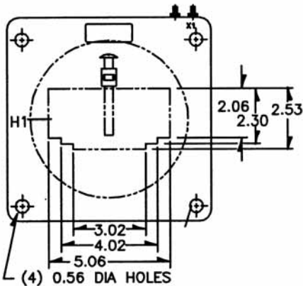
(BUS BAR MOUNTING KIT SHOWN)
